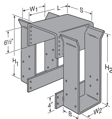
HGLS
