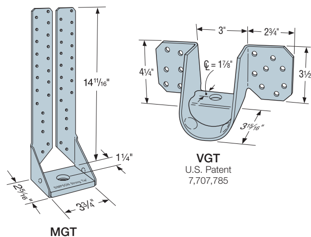
MGT
