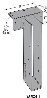
WPU
