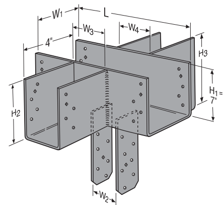
CCCQ-SDS2.5
