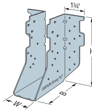
HTU26
