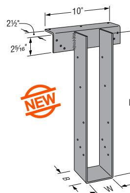
HWP
