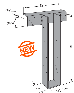
HWPH
