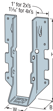
✓ LUS28
