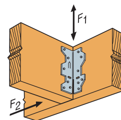
4 A35
