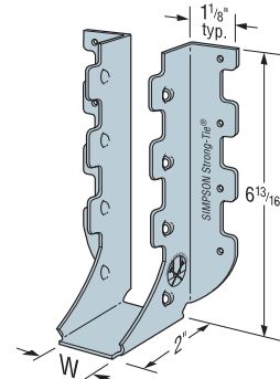
✓ MUS28
