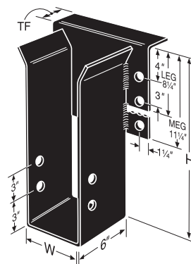
LEGPC/MEGPC
