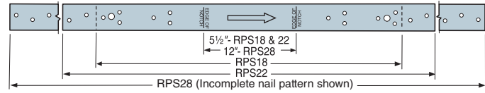
RPS
