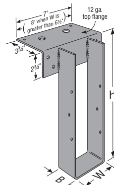
WMU
