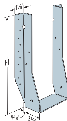
MIU
