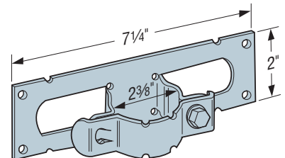
PGT2E
